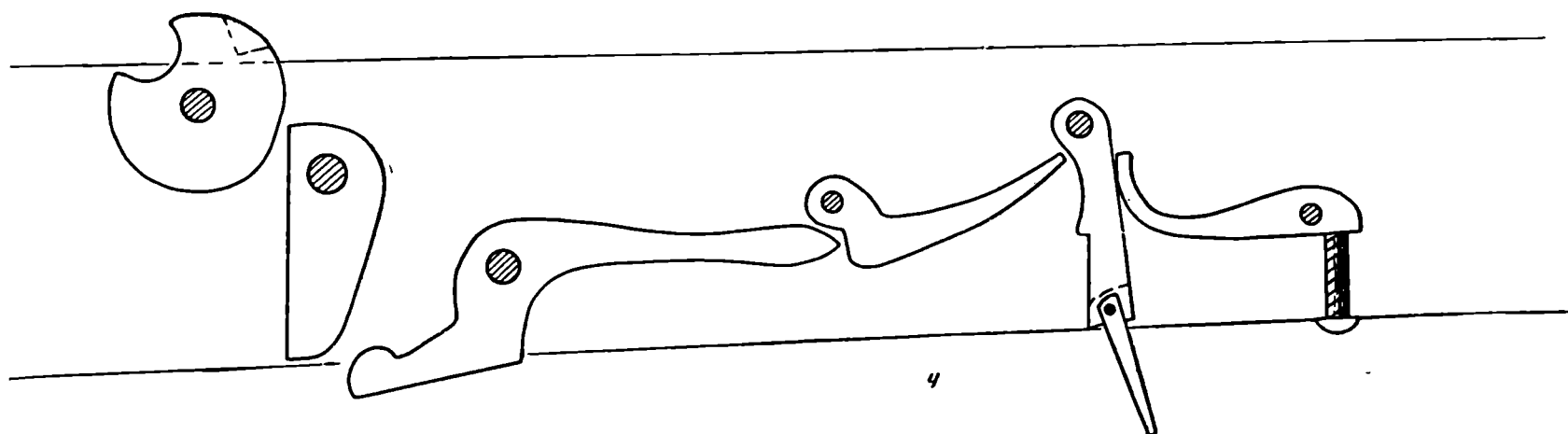
Рис. 5. Самострел. Спусковой механизм 1— вид сверху; 2 — продольный разрез; 3 — на вводе; 4 — после спуска
